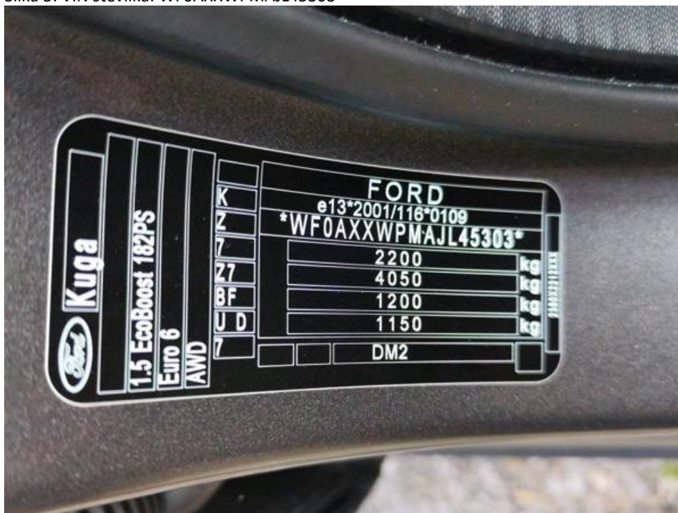
Slika 3: VIN številka: WF0AXXWPM AJL45303
